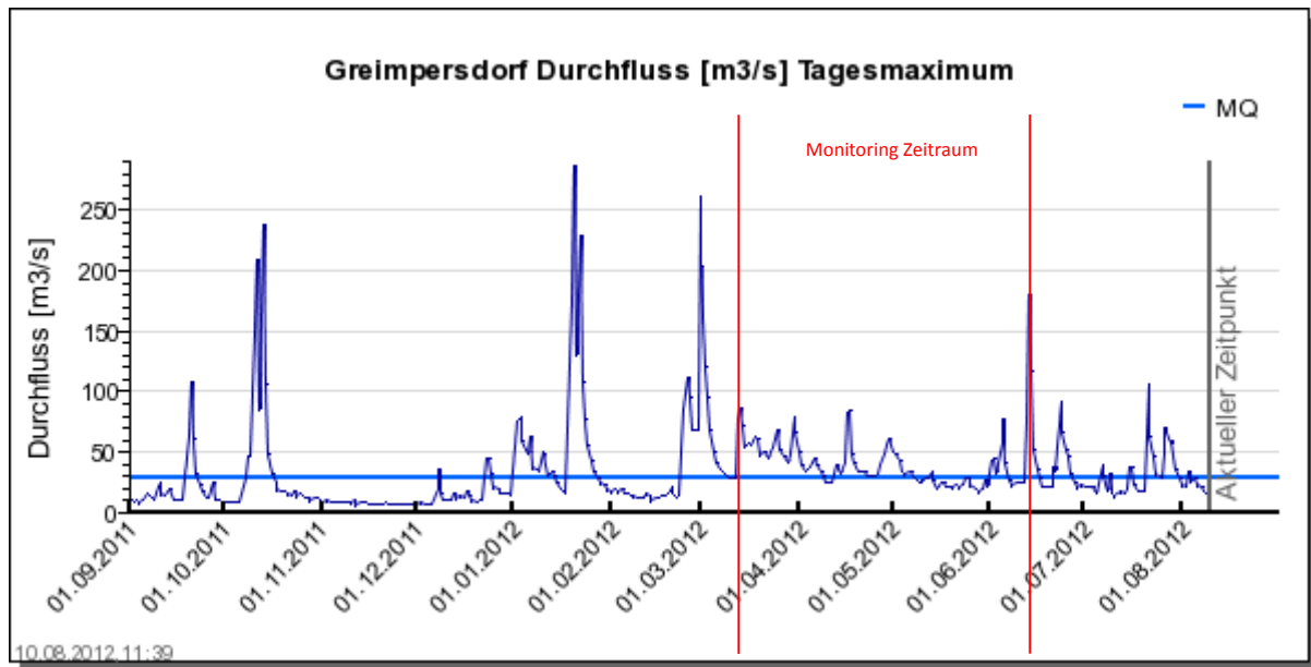
Abb. 6: Durchfluss Ybbs am Pegel Greimpersdorf (www.noel.gv.at, 2012)
