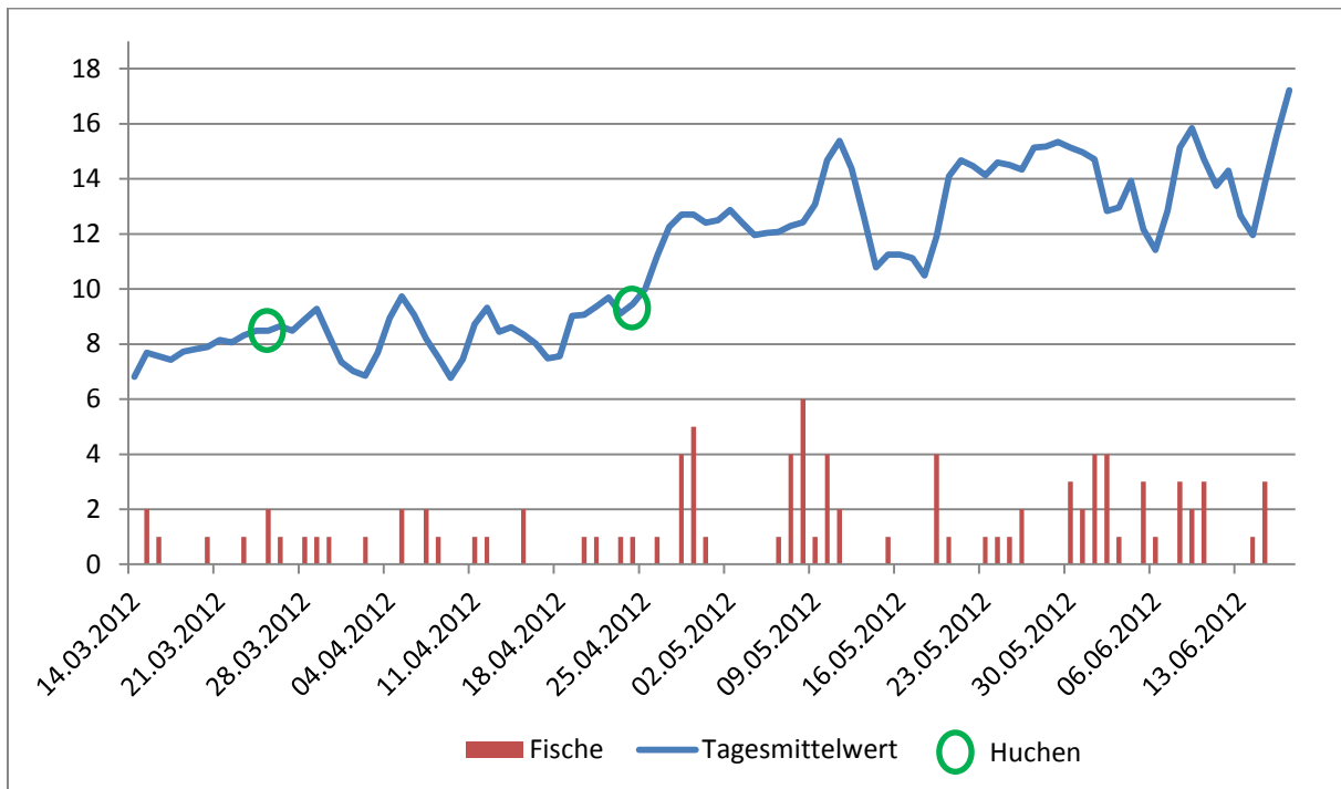
Abb. 14: Temperaturverlauf und Aufstieg der Huchen
