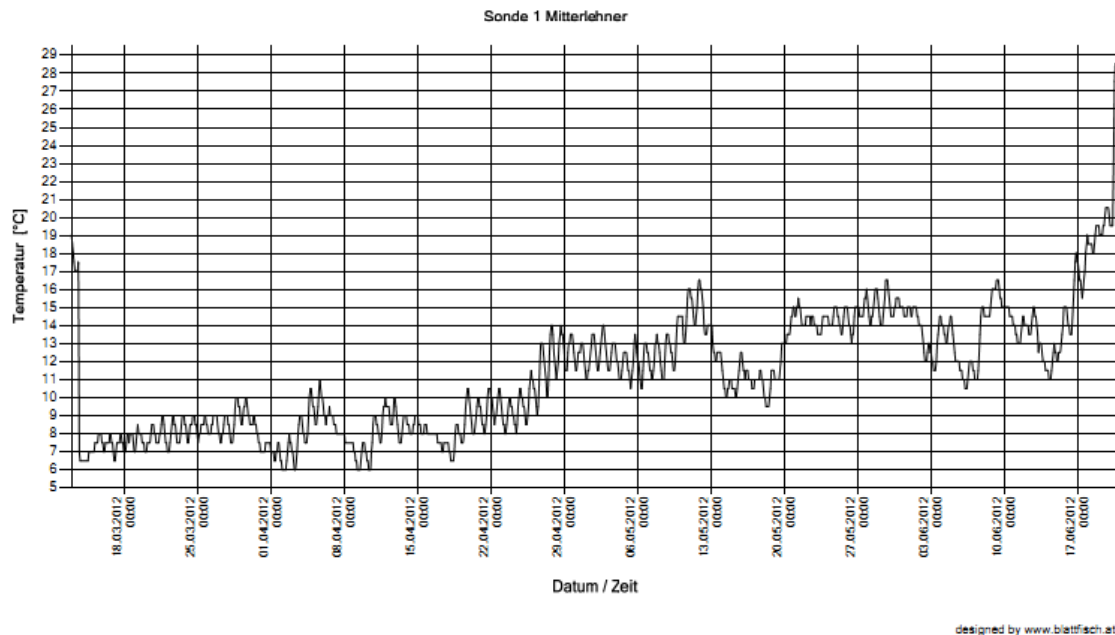
Abb 4. Temperaturdaten Fischwanderhilfe Greinsfurth
