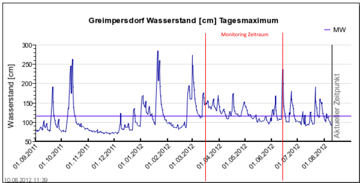
Abb. 7: Wasserstand Ybbs am Pegel Greimpersdorf (www.noel.gv.at, 2012)
