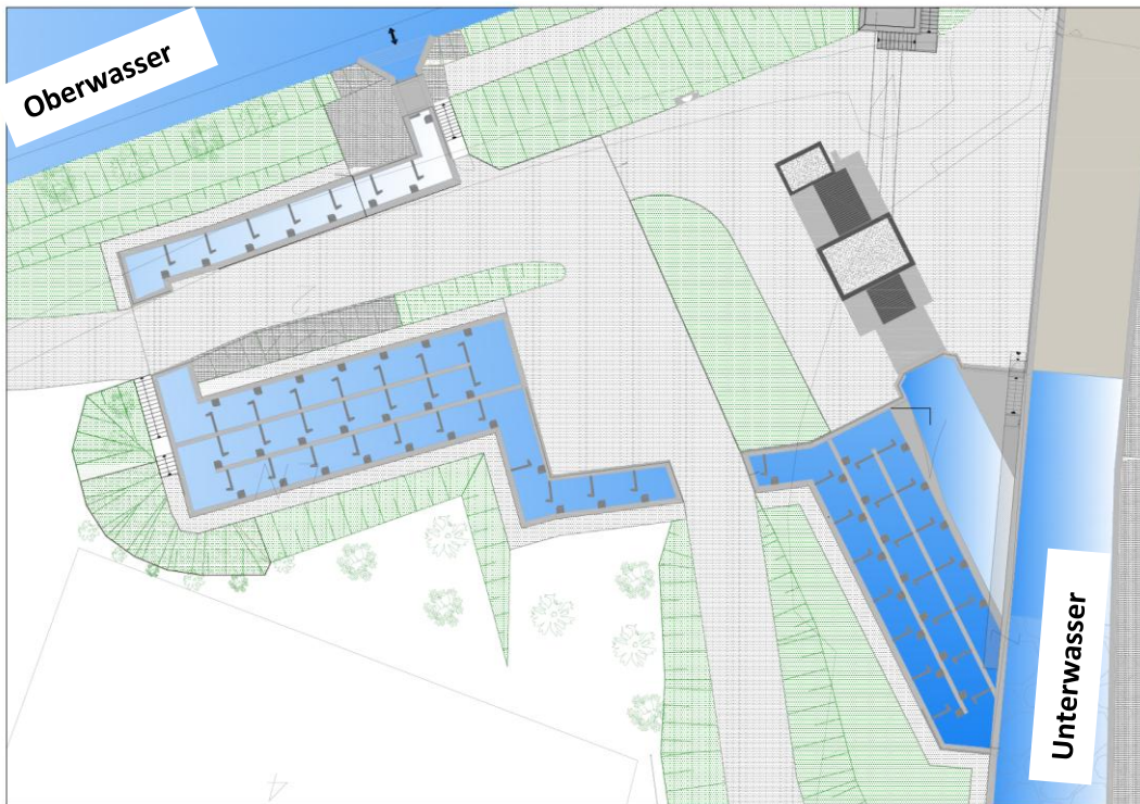
Abb.2: Lageplan
