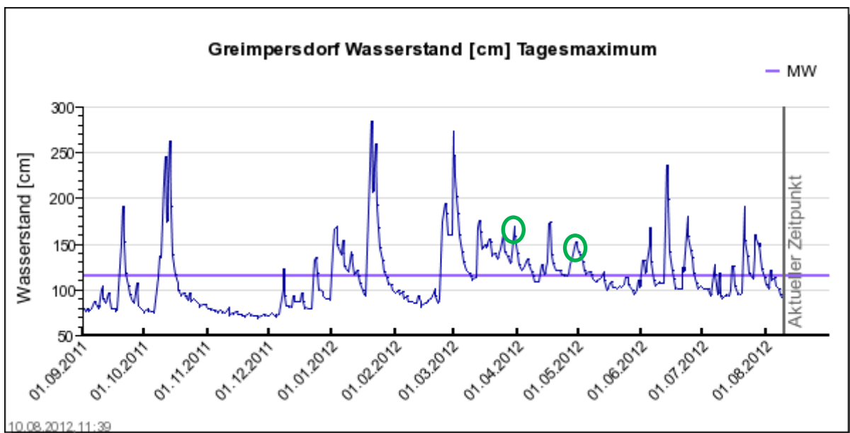
Abb. 15: Wasserstand im Vergleich zu Huchenaufstieg.
