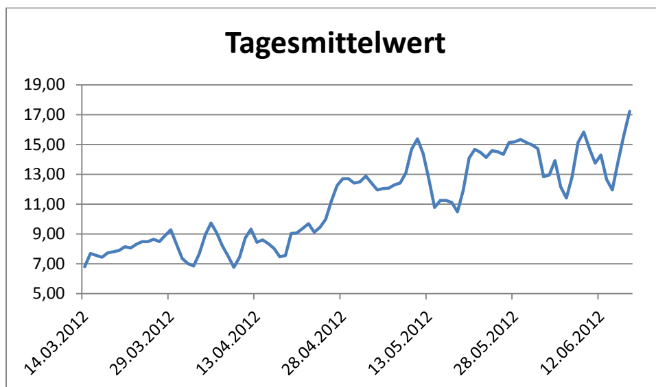
Abb 5: Tagesmittelwerte Temperatur Fischeaufstieg Greinsfurth
